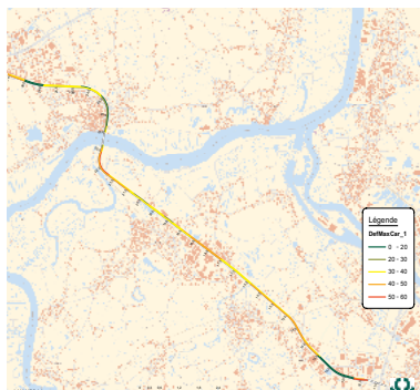
Déflexion maximale caractéristique sur une partie de la N16
